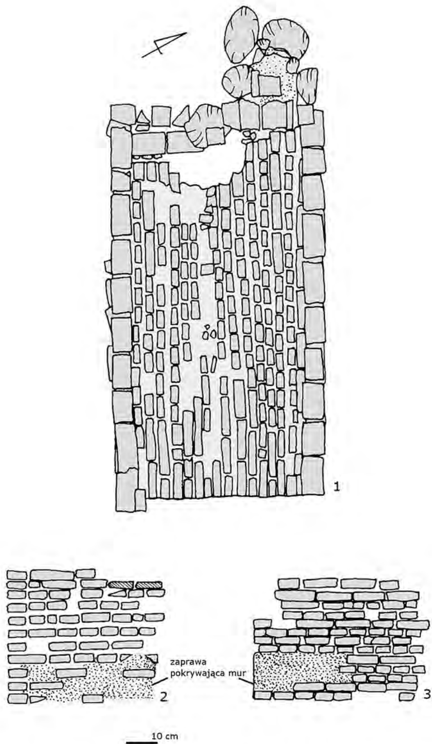
Tablica 2. Białystok, cmentarz ewangelicki przy ul. Młynowej. Grób nr 3 (krypta murowana): 1 – plan sklepienia; 2 – profil ściany północno-zachodniej; 3 – część profilu ściany południowo-zachodniej
