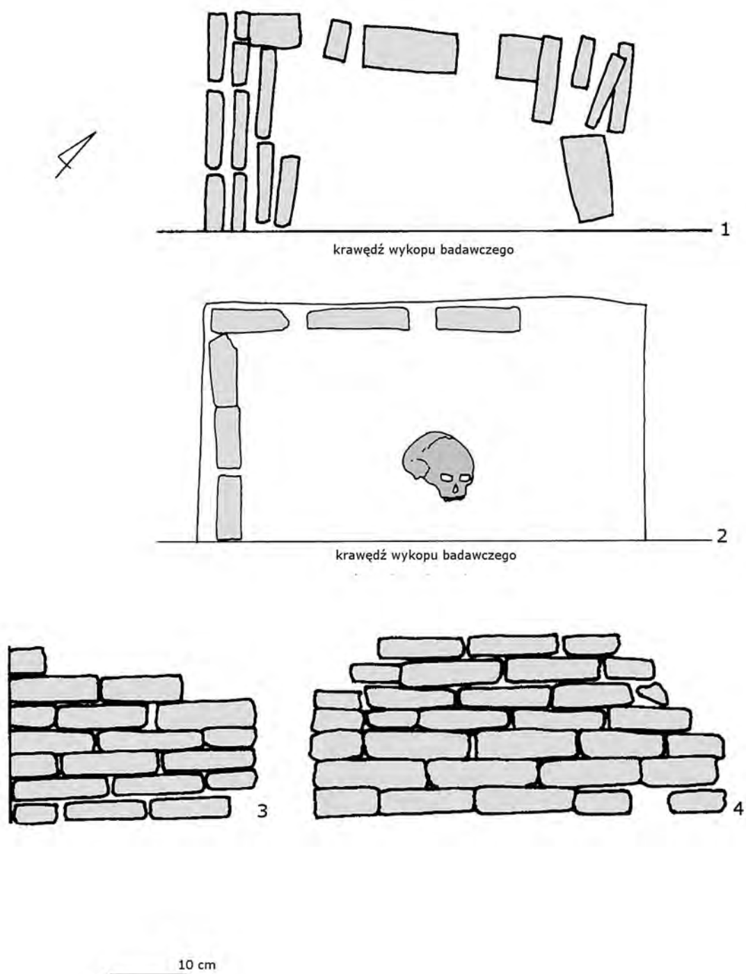
Tablica 1. Białystok, cmentarz ewangelicki przy ul. Młynowej. Grób nr 1 (krypta murowana): 1 – plan zachowanej części sklepienia; 2 – plan na poziomie szkieletu; 3 – profil ściany południowo-wschodniej; 4 – profil ściany północno-zachodniej
