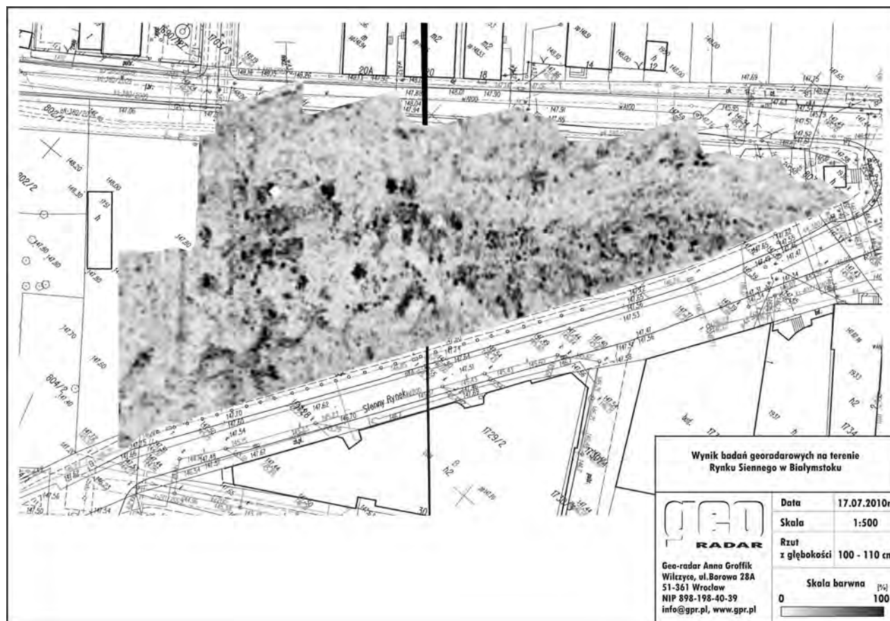
Ryc. 11. Wyniki badań georadarowych. Układy ciemniejszych stref anomalnych wyraźnie odcinających się od tła (jaśniejsze pole). Głębokości 1,00–1,10 m
